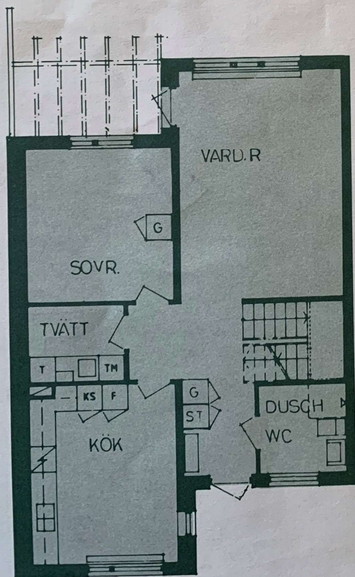
Våning 1
